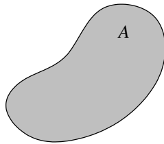
Die Menge A , ...
