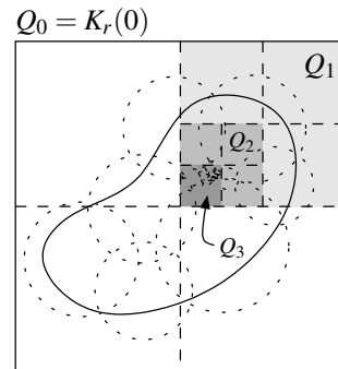
und die Würfel Q_k
