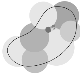
eine offene Überdeckung von A ...
